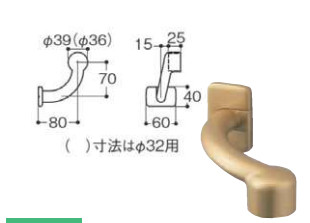
156B-06 出入り口用としてドア近くの握りやすい位置に手すりを取り付けすることができます。 ④21262 オフセットブラケット(上下一組)
