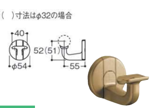
156B-07 墨出しの際、木棒中心位置にブラケットをあわせるだけで施工が簡単です。 ④21328 L付受ブラケット
