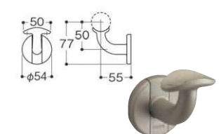
156B-08 支持部が下方に逃げているので、手を離さずに伝うことができます。 ④21025 L付受ブラケット
