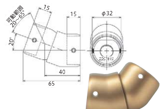
156B-13 20°から65°の間で自由に曲げられます。 ④21043 フレキシブルジョイント
