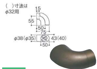
156B-04 さまざまなシーンに適したシンプルなデザインです。 ④21034 エンドホルダー
