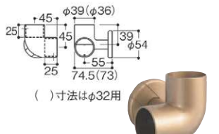
156B-11 縦手すりと横手すりを90°に取付けることができます。 ④22673 コーナーブラケット
