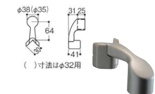
156B-09 柱などの出隅部分に縦手すりを取り付けることができます。 ④21037 出隅ブラケット
