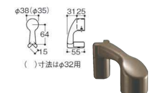
156B-10 壁固定部の受け面が狭いので、ドア縁にも取付けることができます。 ④21288 出隅スリムブラケット
